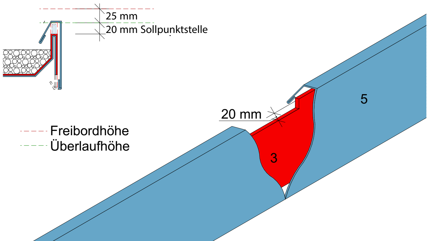
Abb. 42: Sollpunktstelle (Beispiel 4)
