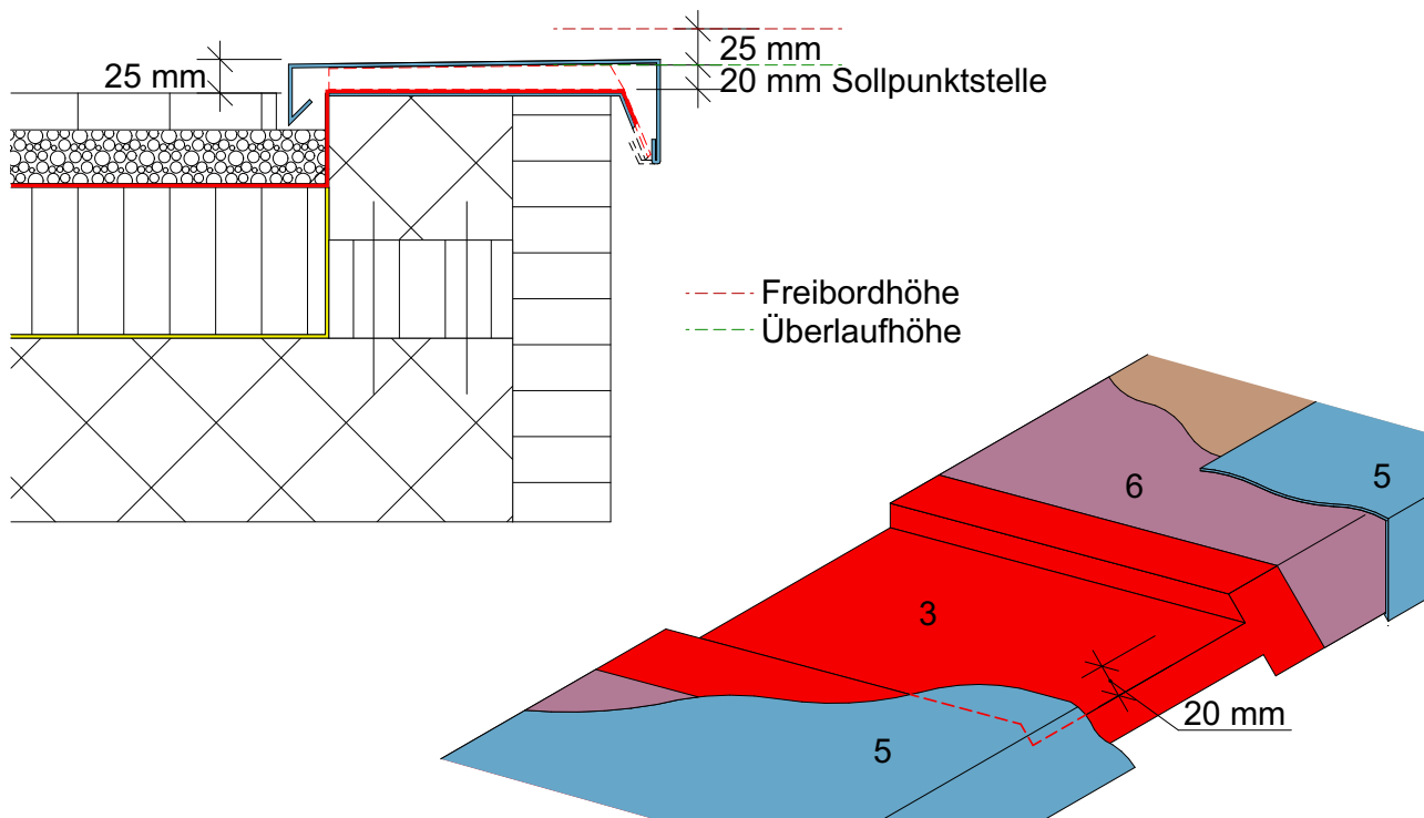
Abb. 41: Sollpunktstelle (Beispiel 1)
