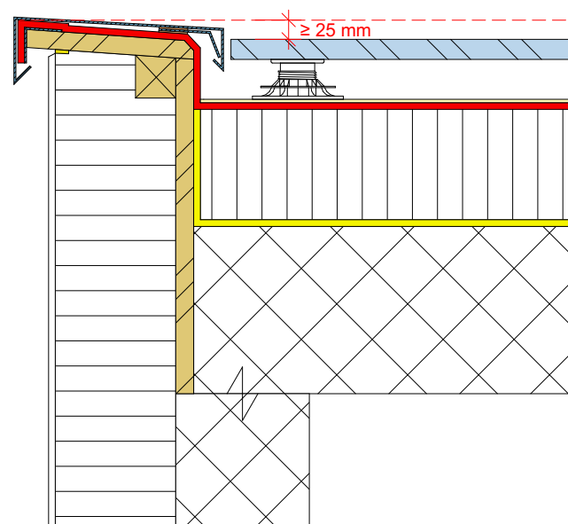
Abb. 28: Überlaufsicherer Dachrand muss mindestens 25 mm über der Schutz- und Nutzschicht geführt werden. Norm SIA 271:2021 Art. 2.8.1.6 Figur 8
