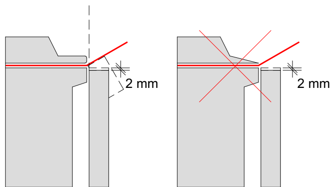
Abb. 19: Biegewange mindestens 2 mm tiefer einstellen und die Rundschiene einsetzen
