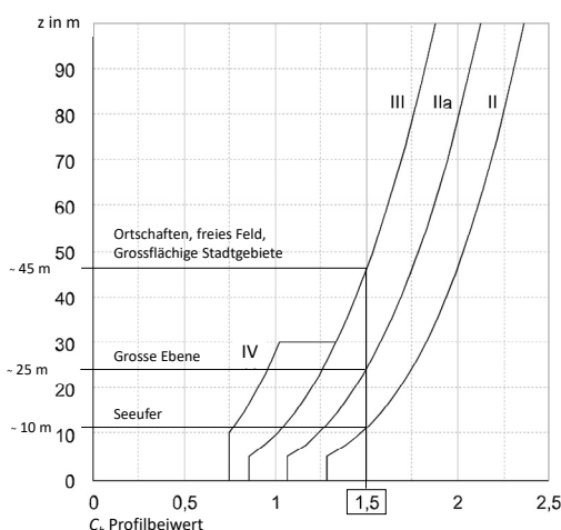
Abb. 3: Profilbeiwert c_p in Abhängigkeit von der Höhe z Quelle: SIA 261 Figur 6
