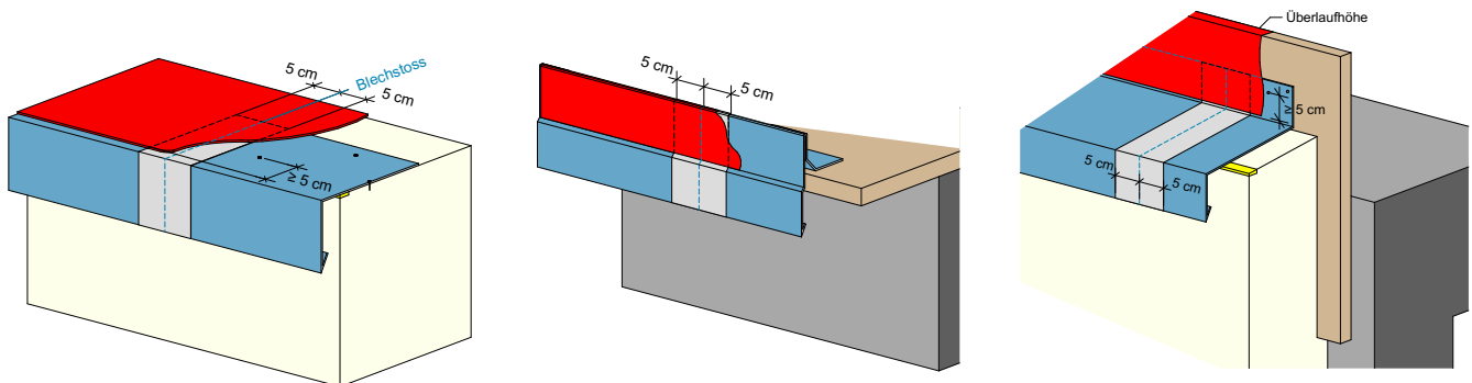
Abb. 10: Ausbildung der Blechstöße bei überlaufsicheren Dachrandkonstruktionen
