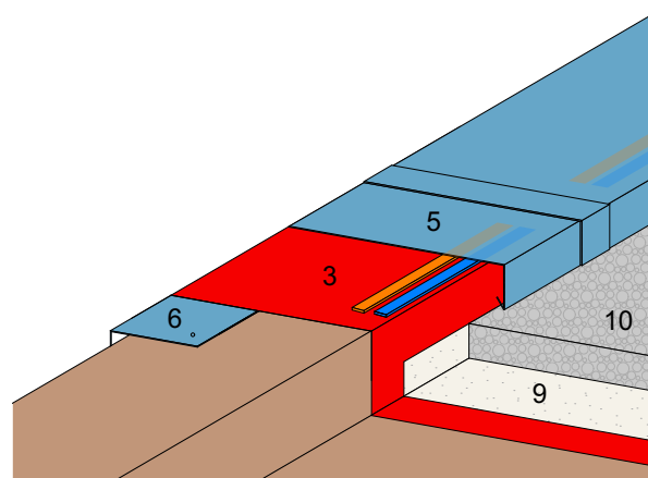
Abb. 21: Dachrand Kleberauftrag
