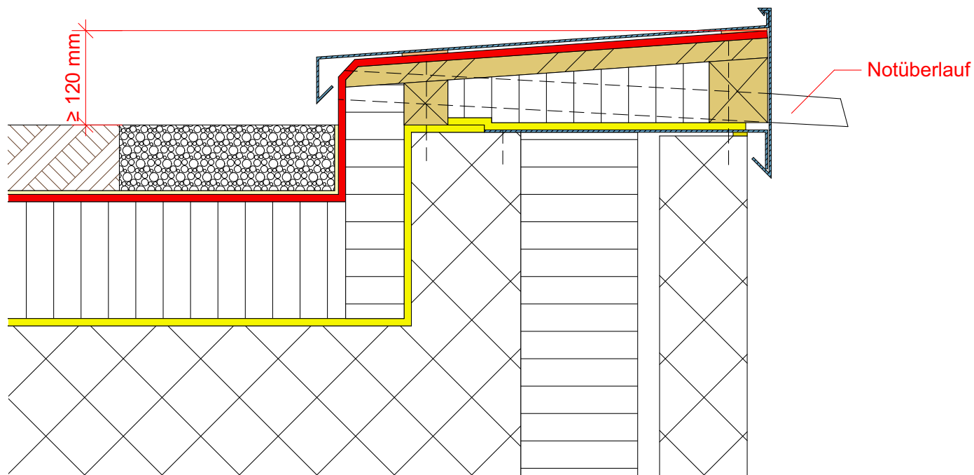
Abb. 31: Nicht überlaufsichere Dachrandkonstruktionen (Beispiel 2, Sanierungslösung)
