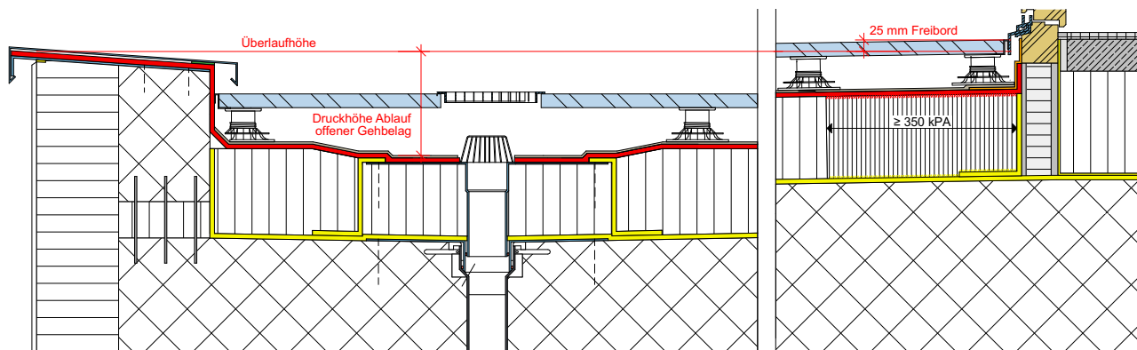
Abb. 7: Oben offener Gehbelag
