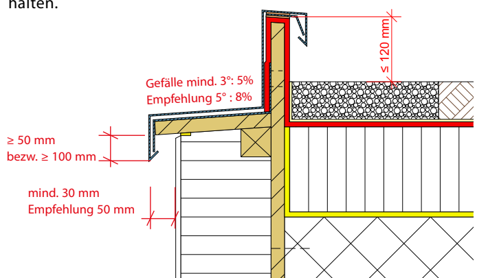
Abb. 5: Dachrandabschluss, Entwässerung nach Aussen
